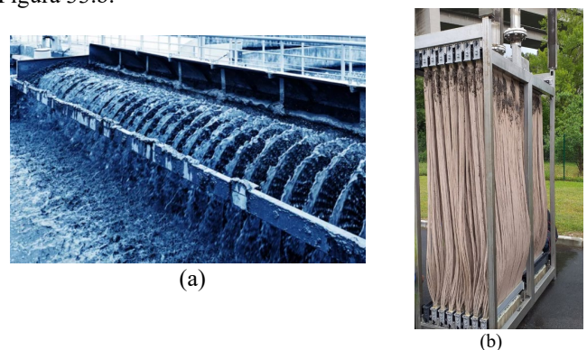
Figura 33 Sistema de biodiscos (a), Membranas en interior de biorreactor aireado (b).
