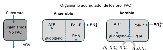
Figura 23. Proceso básico de la eliminación biológica de fósforo
