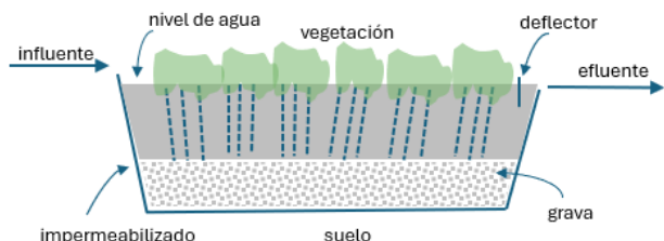
Figura 5. Esquema de humedal de flujo superficial
