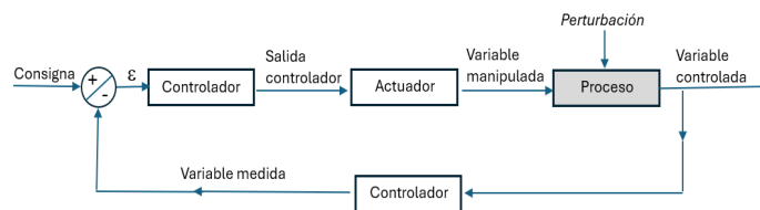
Figura 43. Esquema de un proceso tradicional de control con retroalimentación.
