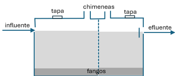
Figura 4. Esquema de fosa séptica
