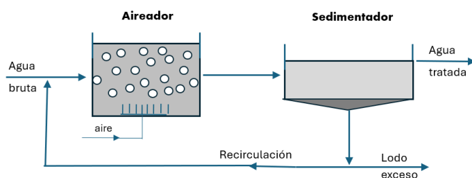
Figura 26 .Esquema básico de lodos activados
