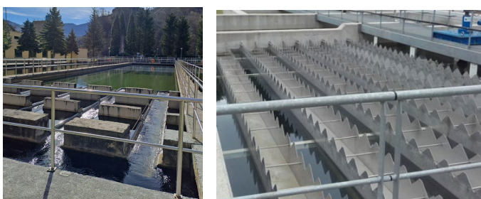
Figura 10. Decantador y Separación en lecho de filtración (desarenado)
