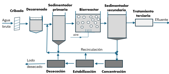
Fig. 31. Diagrama de una planta EDAR
