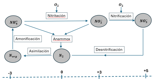
Figura 23 Transformaciones básicas interesantes de nitrógeno y estados de oxidación
