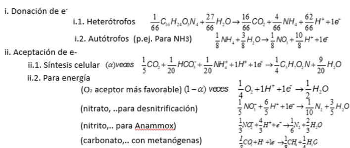
Figura 22 Elaboración de la estequiometría para procesos biológicos de tratamiento de aguas
