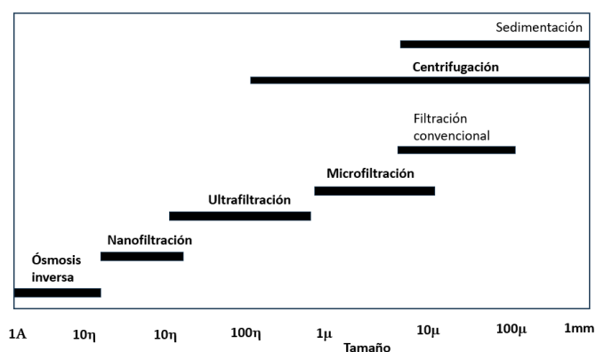
Figura 24. Intervalos de separación con procesos de separación de velocidad y de filtración
