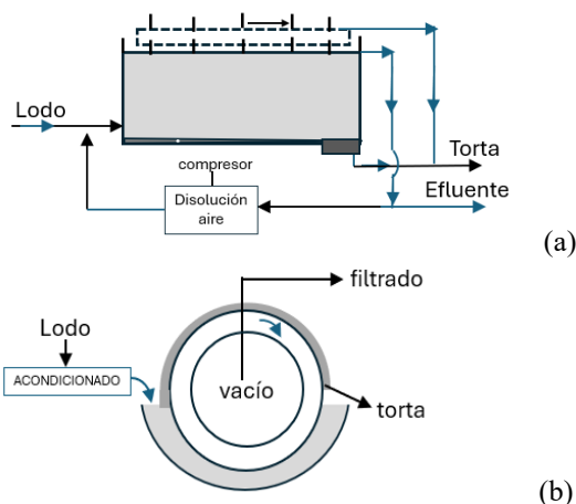
Figura 37. Esquema de dos equipos en la concentración de fangos: (a) Flotación y (b) Filtración a vacío
