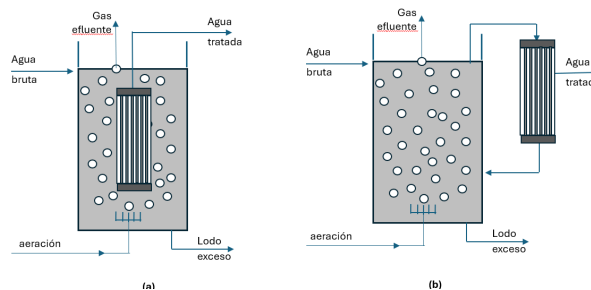
Figura 25. Biorreactores de membrana; (a) membrana sumergida, (b) membrana externa
