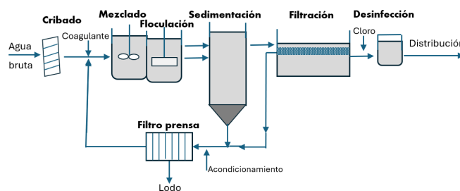
Figura 7. Esquema general de una planta ETAP
