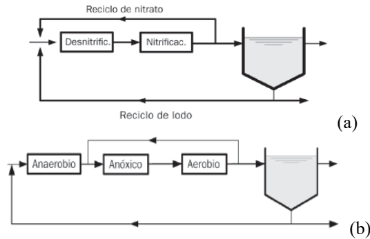
Figura 27 (a) Proceso de eliminación de C y N con desnitrificación a la entrada, (b) Ejemplo de un proceso de eliminación de C, N, P (proceso A2/O)
