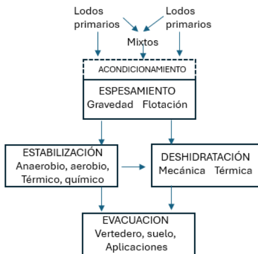
Figura 36. Etapas en el tratamiento de lodos
