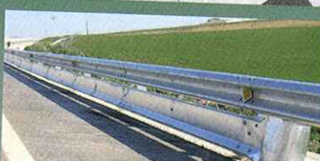
Barrera Metálica con Sistema de Protección para Motociclistas SPM
