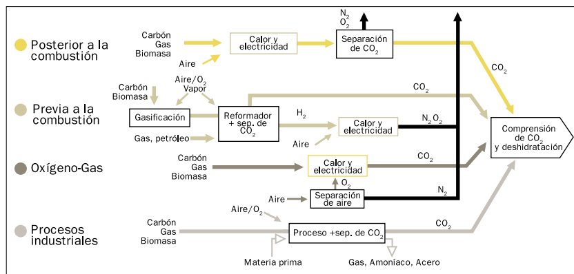
Figura 3. Los sistemas de captura de CO 2 (IPCC, 2005).
